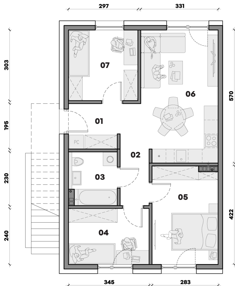
RZUT PARTERU
