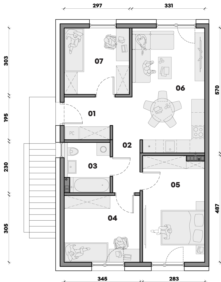
RZUT PIĘTRA
