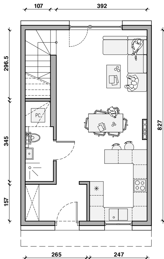
RZUT PARTERU
