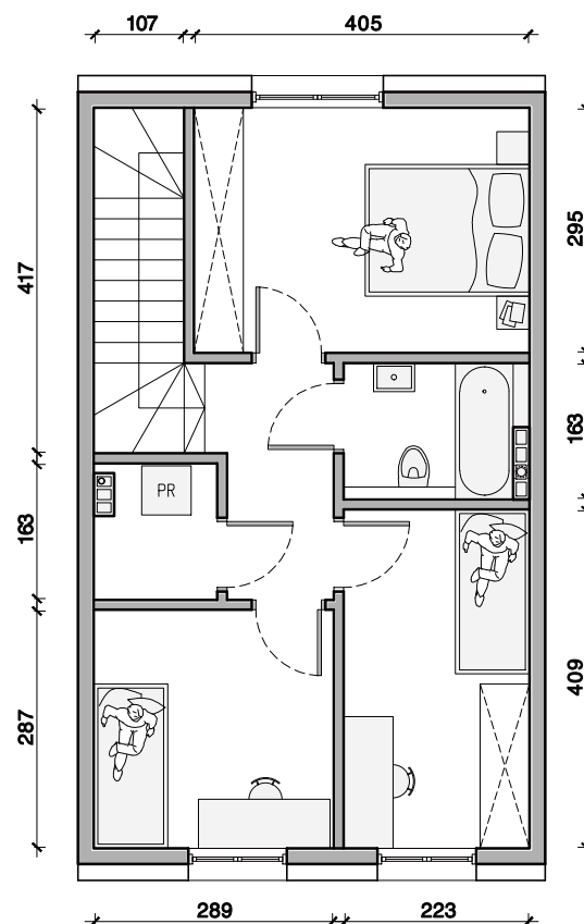
RZUT PIĘTRA
