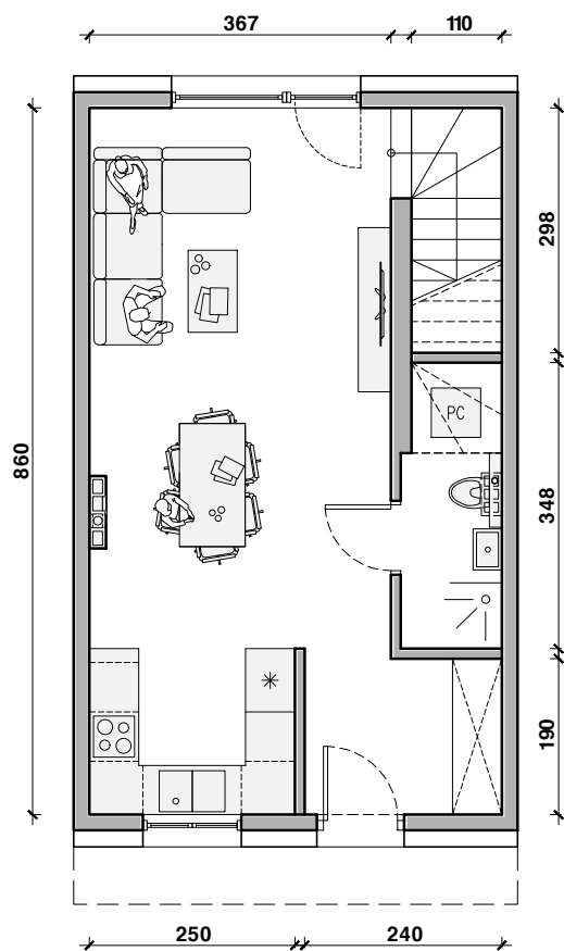
RZUT PARTERU
