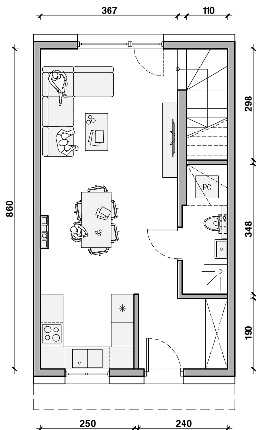
RZUT PARTERU
